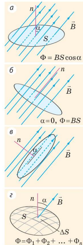
Рис. 13.1. До визначення магнітного потоку
